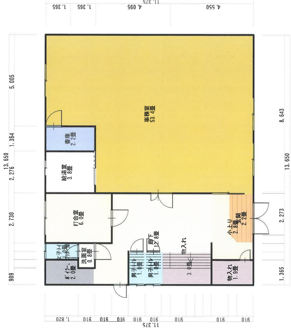
1階縮尺 1/100
